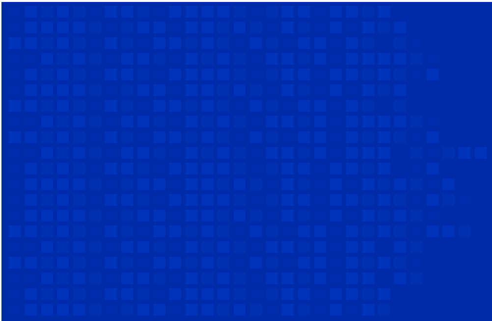
Red celular
